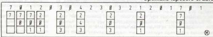
Optimális lappcere 5. ábra
